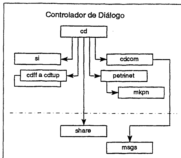
Figura 2: Composição do Controlador de Diálogo
