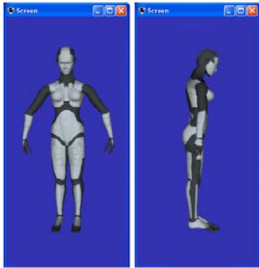
Figure 7: Emoción Tristeza
