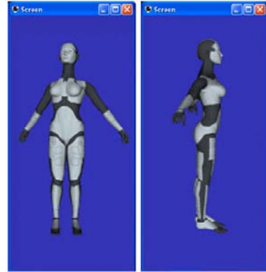
Figure 5: Emoción Alegría
