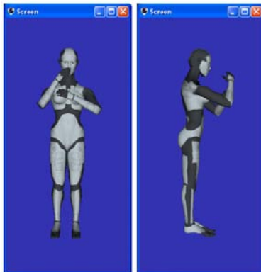
Figure 4: Emoción Miedo
