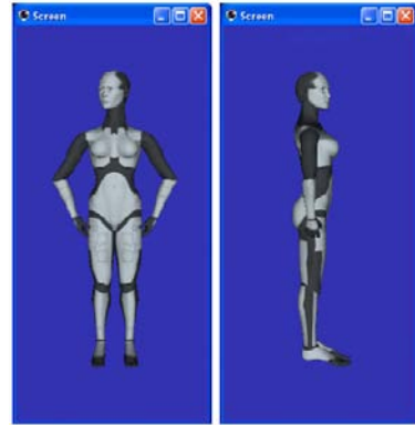
Figure 6: Emoción Aversión
